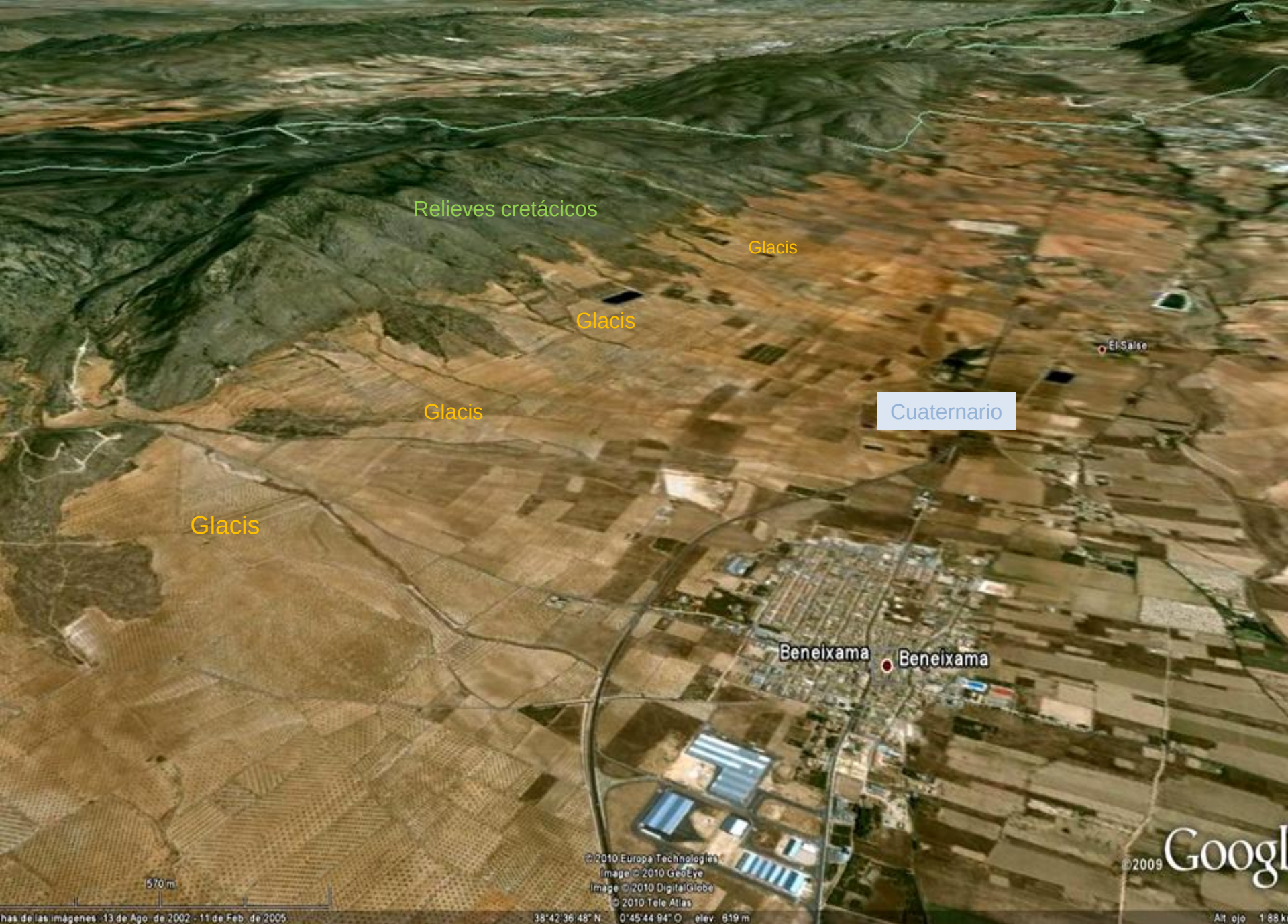
Relieves cretácicos con numerosos pliegues y fallas de orientación Bética. Glacis Cuaternario
