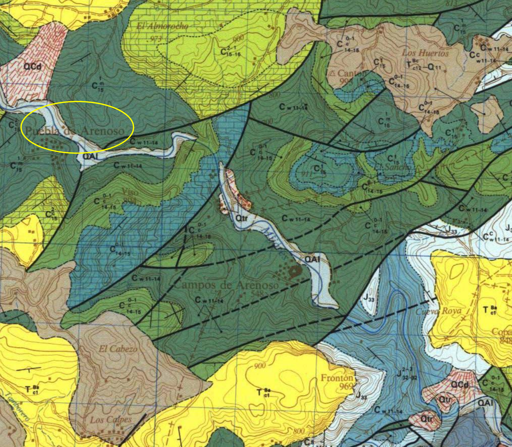
Fragmento del Mapa Geológico 1:50.000 -614 – Manzanera. Sin representación del Embalse
